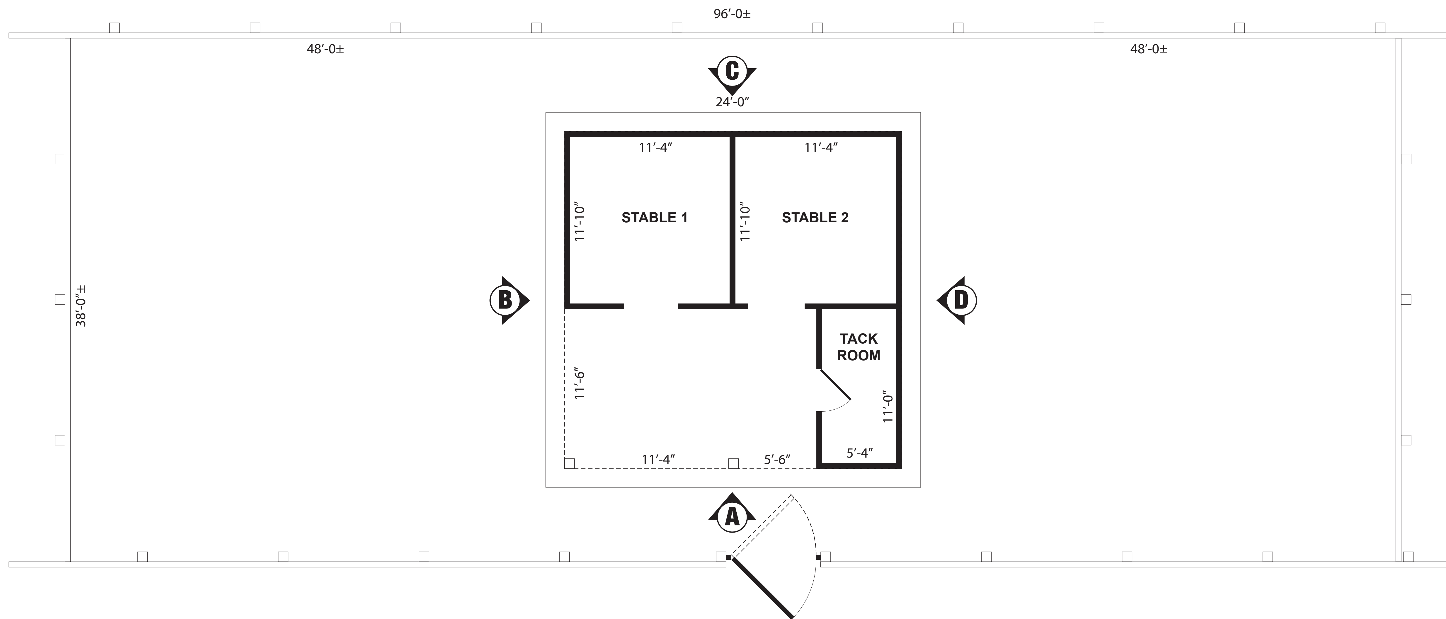
PADDOCK PLAN
