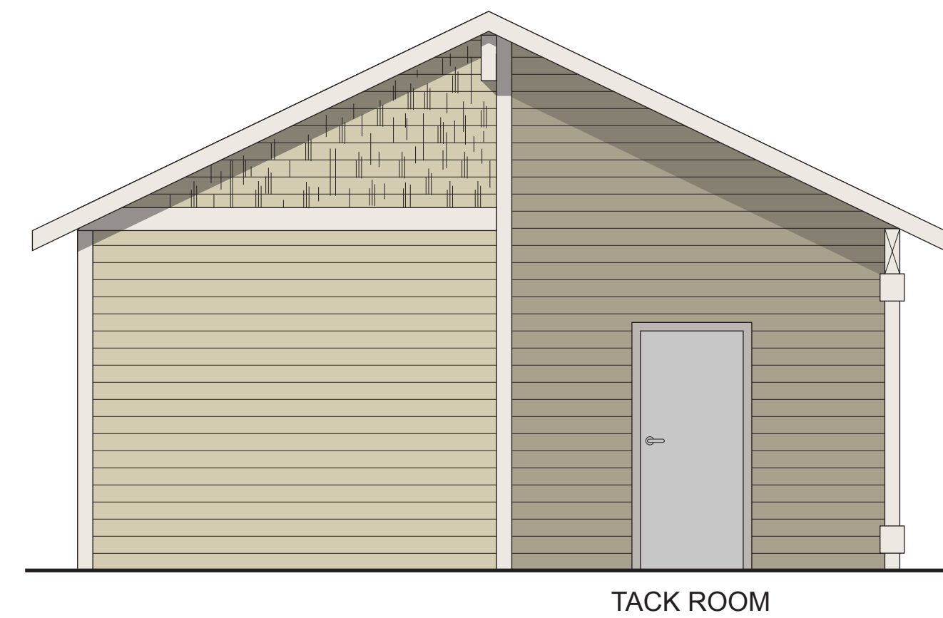
ELEVATION B
